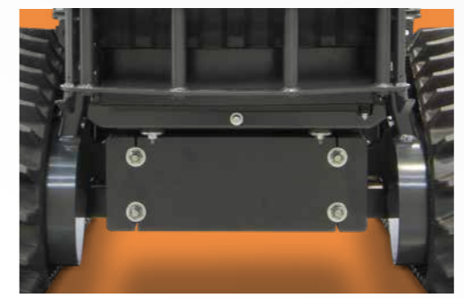
Zavorre aggiuntive da 70 Kg Additional 70-kg ballasts
